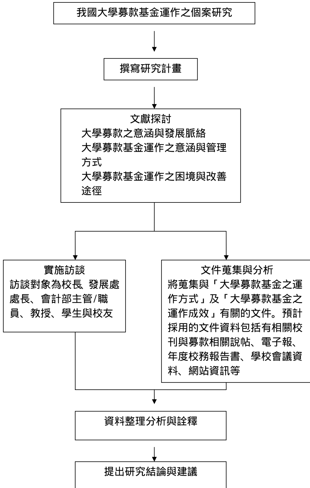
圖1-1 研究流程圖
