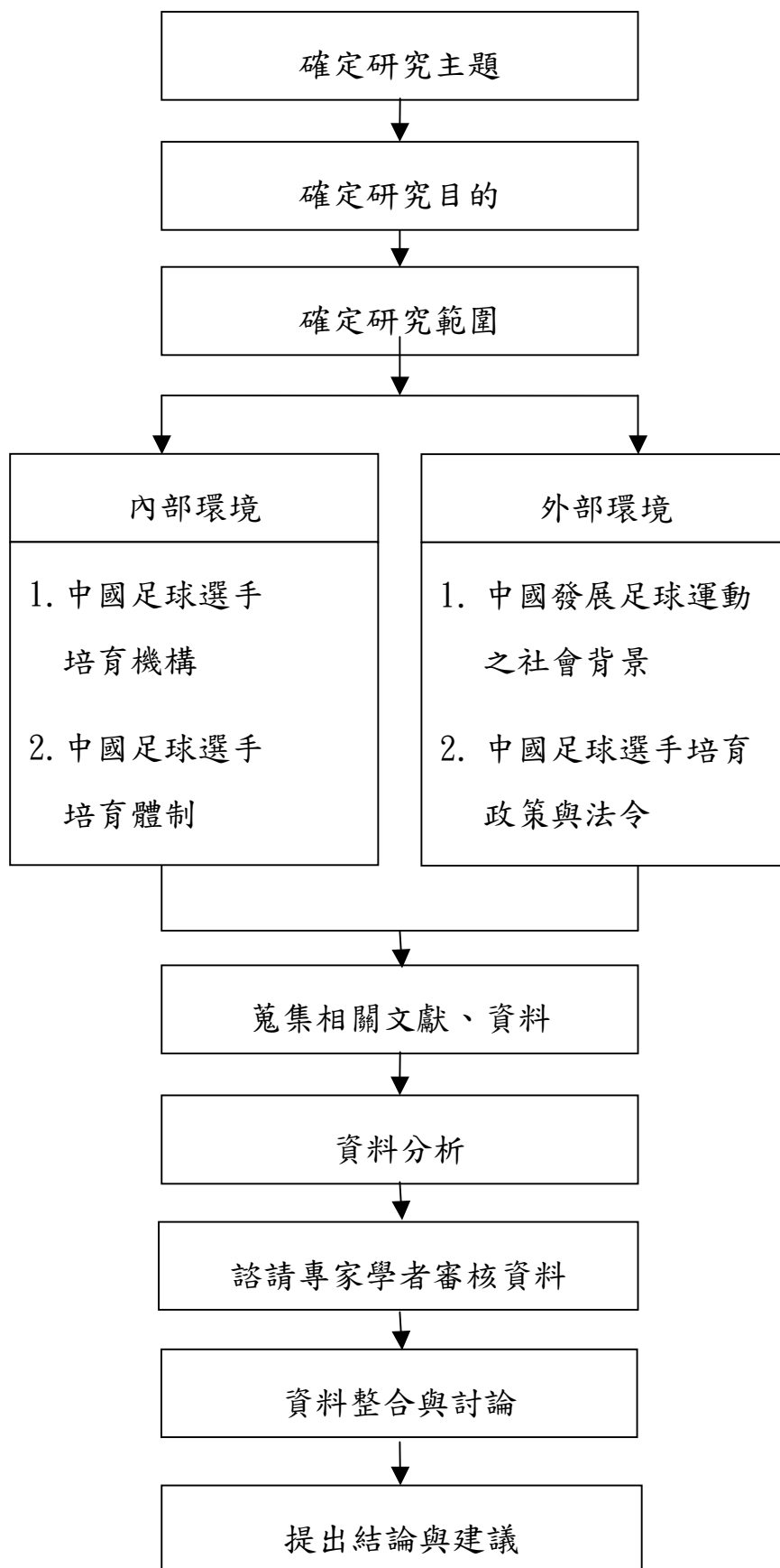
圖 3-2-1 研究流程圖
