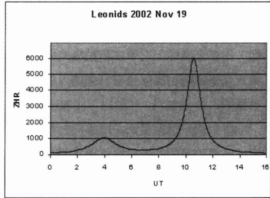
圖八 1998 年與 2002 年獅子座流星雨天頂流星數量
