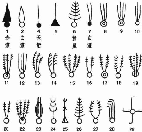
圖四 馬王堆出土白絹上的各式彗星
