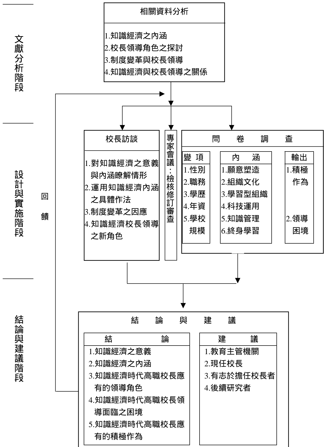
圖 3-1 研究架構圖
