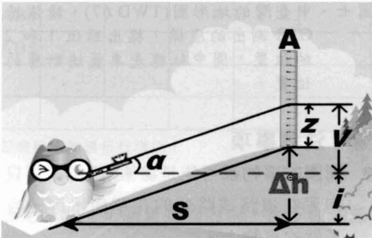
圖八、三角高程測量法：灰色框表示手水準儀，黃色杆子表示標尺，S 是水平距離，Δh 是相對高度，α 是投影出來的角度，有了這些，只要沿著地形切面重複使用三角高程測量法測量高度，就可以繪出你們要的剖面圖。
