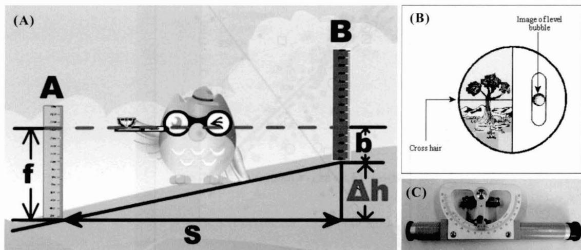
圖六、(A)水平標高測量法於地形剖面之示意圖：灰色器具代表手持水準儀，黃色杆子表示標尺，S 表示標尺 A 和 B 的水平距離，f 是標尺 A 從地表到手持水準儀上觀察到的高度數值，b 則是地表到手持水準儀，用標尺 B 測量觀察到的高度數值，用 f 減掉 b 得到的 \Delta h ，就是 A 和 B 的相對高度差。(B)手持水準儀觀測視窗示意圖，右半邊為水平儀。當氣泡置中時代表平視，左半邊為測量觀測窗，其中黑線為視線高度。(C)手持水準儀照片。
