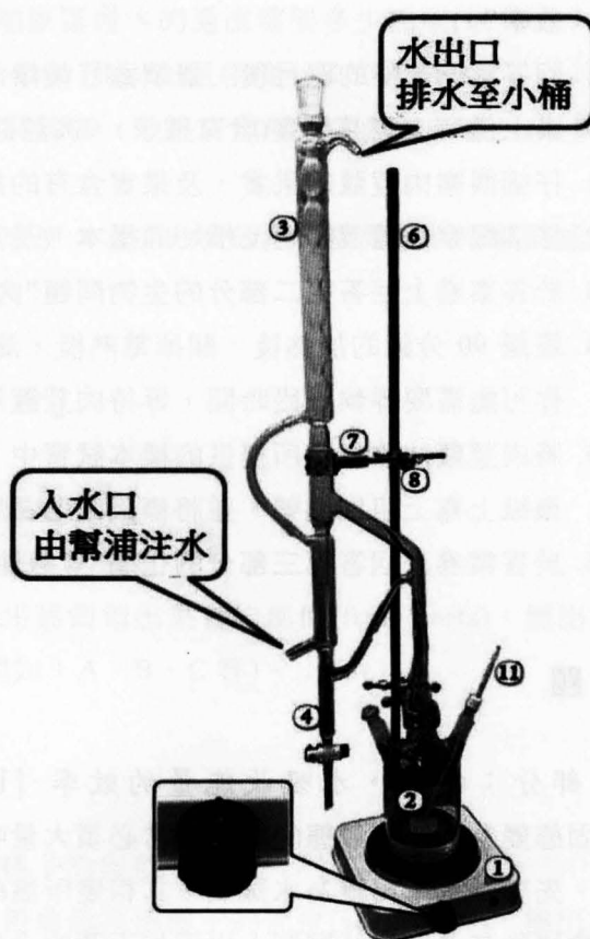
圖 1、水蒸餾裝置，用於分離肉豆蔻油與肉豆蔻籽
