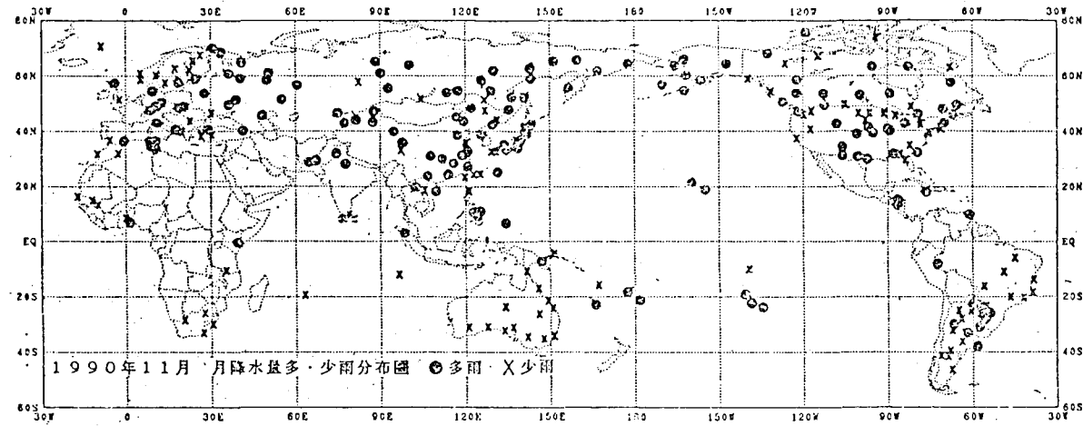
圖3.11 1990年11月月降水量多、少分布圖
