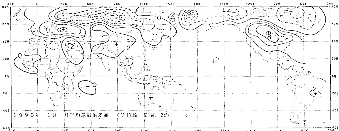
圖2.1 1990年1月月平均氣溫偏差圖
