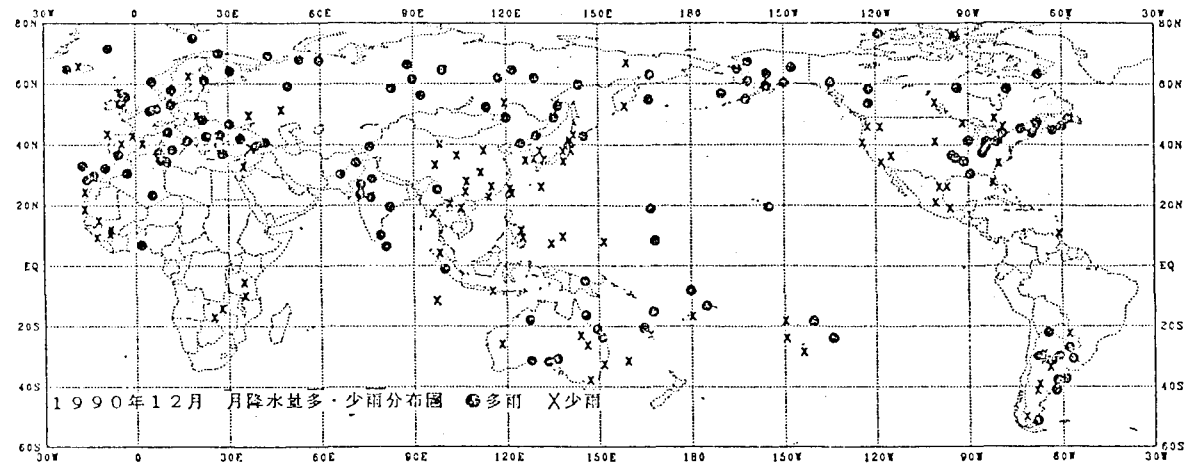
圖3.12 1990年12月月降水量多、少分布圖
