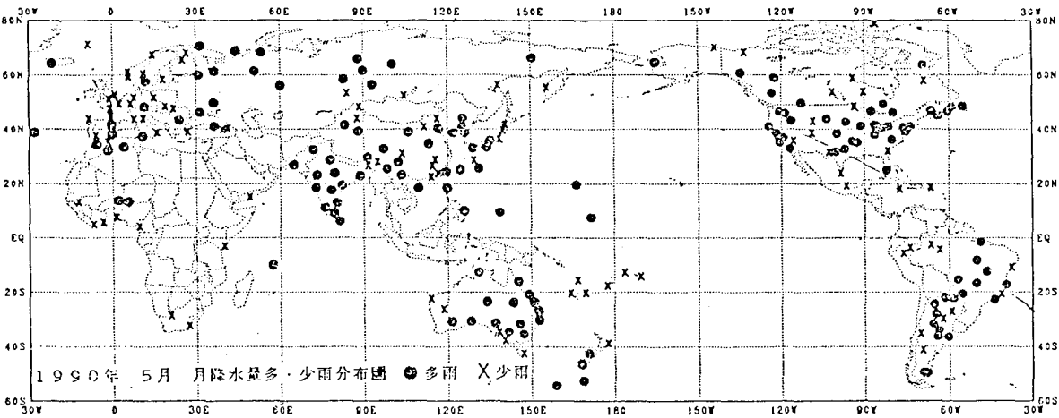
圖3.5 1990年5月月降水量多、少分布圖
