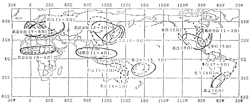
圖 1 1990 年世界主要異常天候
