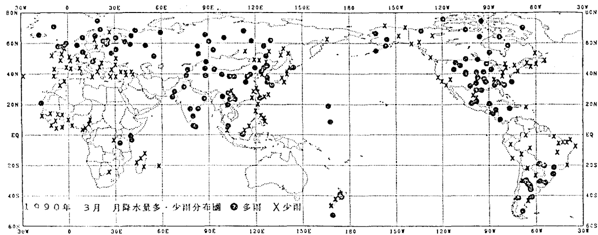
圖3.3 1990年3月月降水量多、少分布圖
