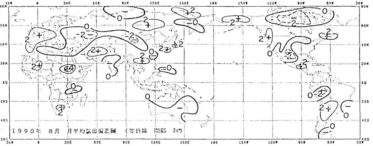
圖2.8 1990年8月月平均氣溫偏差圖
