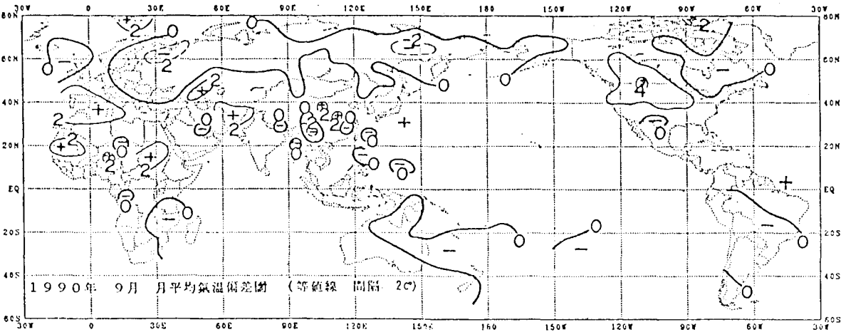
圖2.9 1990年9月月平均氣溫偏差圖
