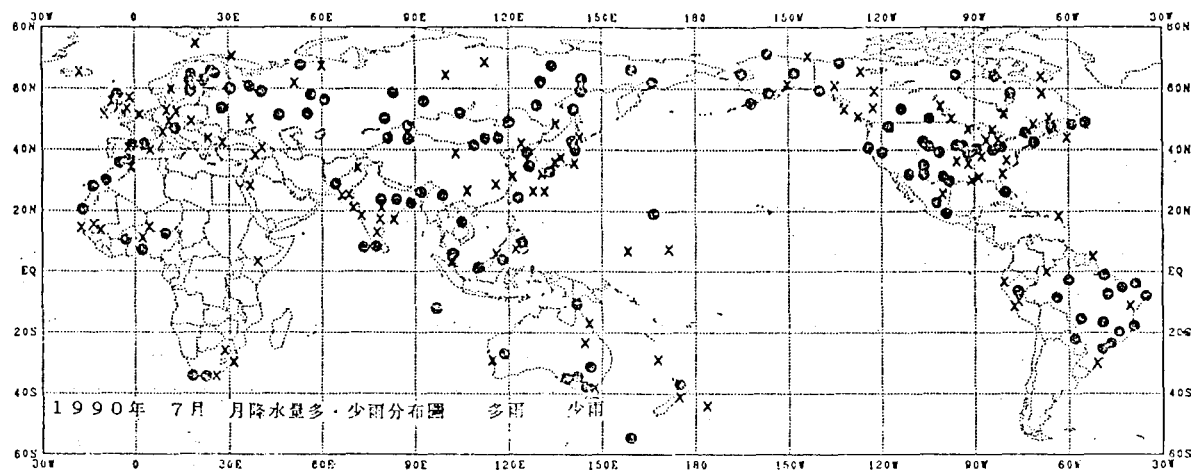
圖3.7 1990年7月月降水量多、少分布圖
