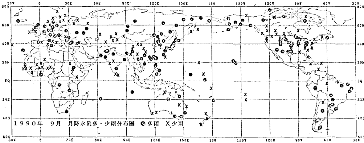
圖3.9 1990年9月月降水量多、少分布圖
