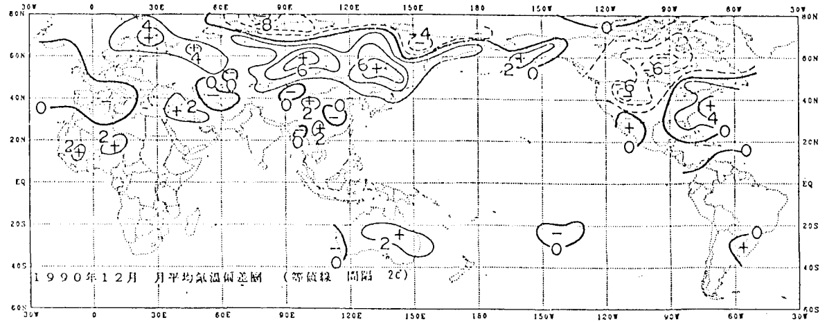
圖2.12 1990年12月月平均氣溫偏差圖
