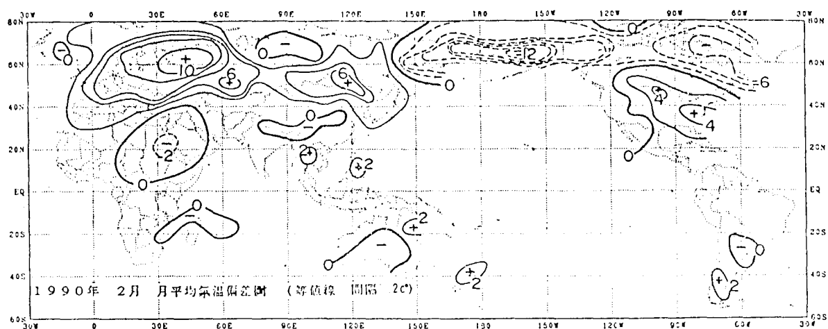
圖2.2 1990年2月月平均氣溫偏差圖
