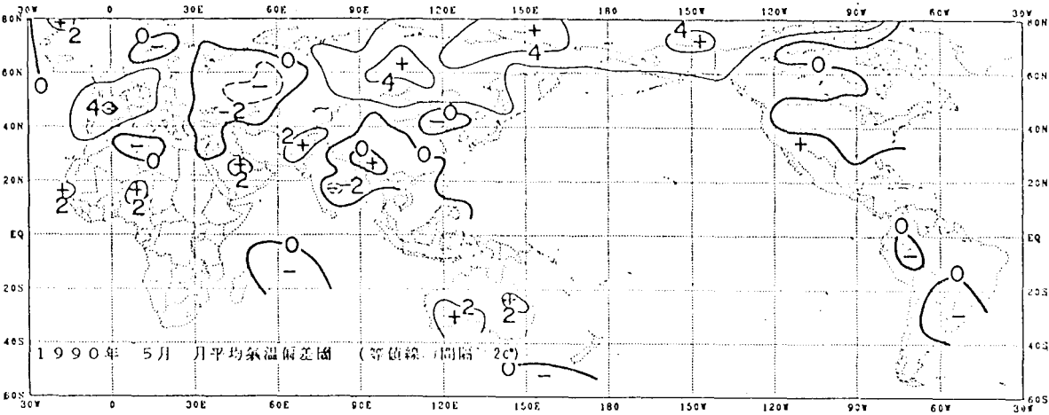
圖2.5 1990年5月月平均氣溫偏差圖
