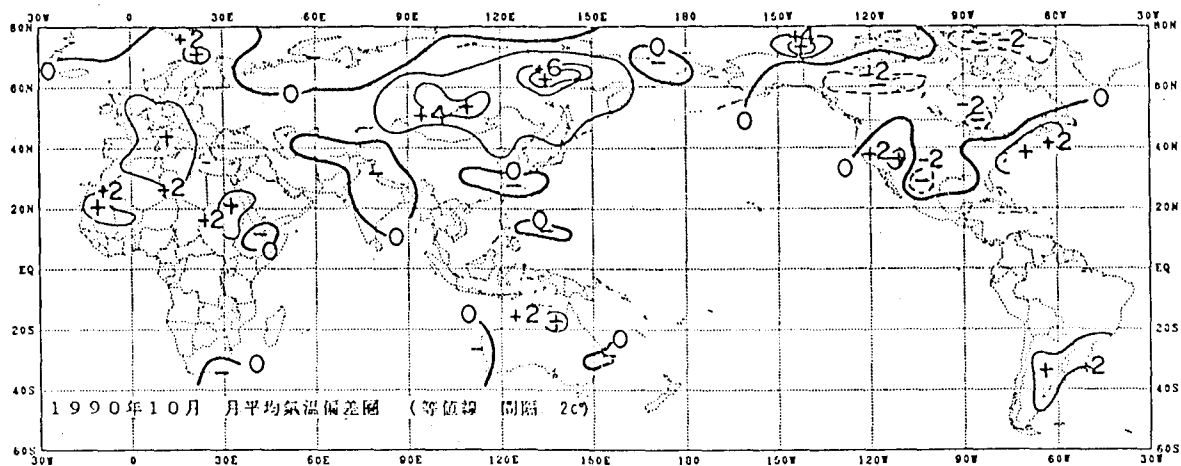
圖2.10 1990年10月月平均氣溫偏差圖
