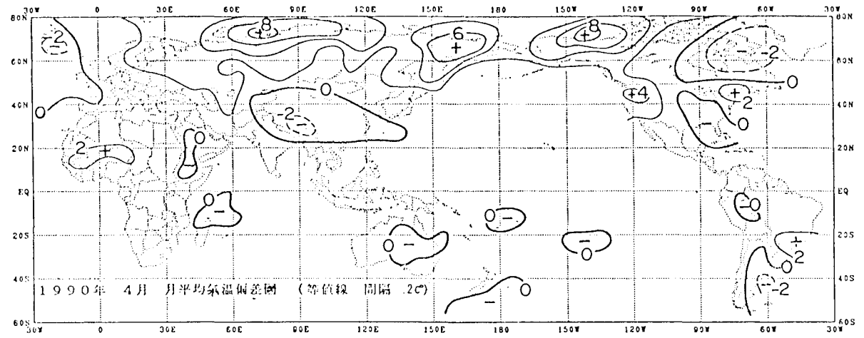
圖2.4 1990年4月月平均氣溫偏差圖
