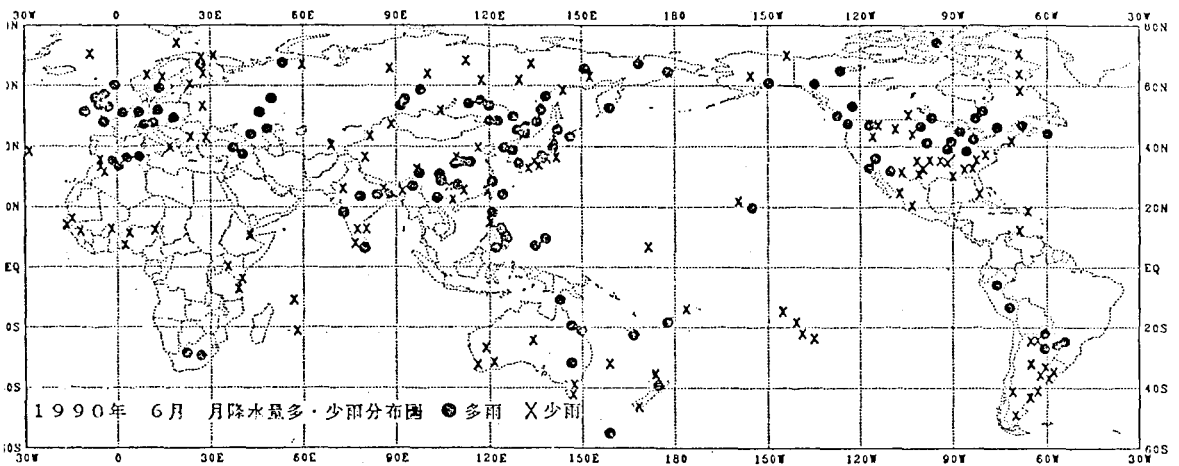
圖3.6 1990年6月月降水量多、少分布圖
