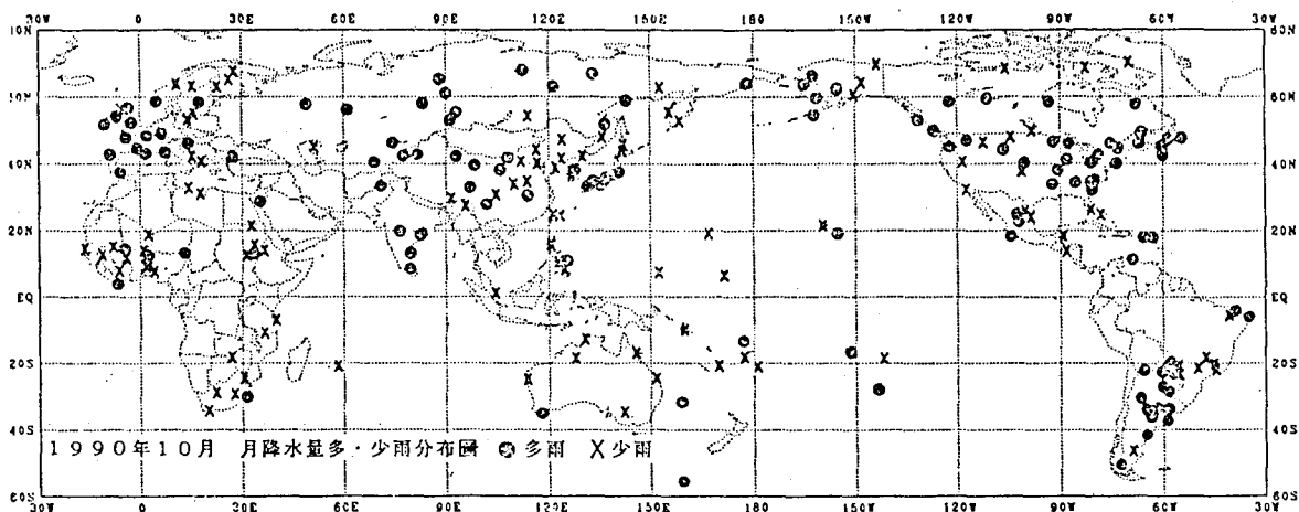
圖3.10 1990年10月月降水量多、少分布圖
