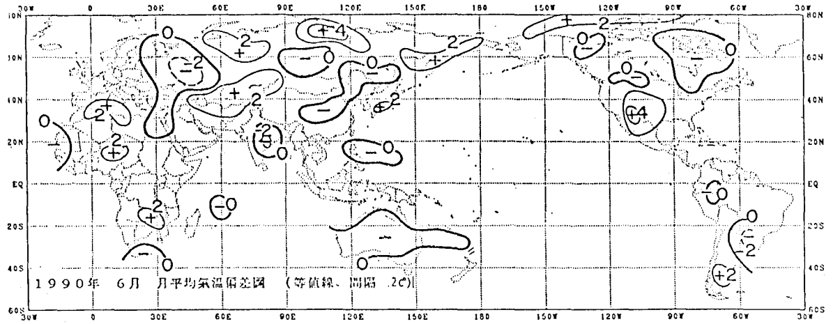
圖2.6 1990年6月月平均氣溫偏差圖
