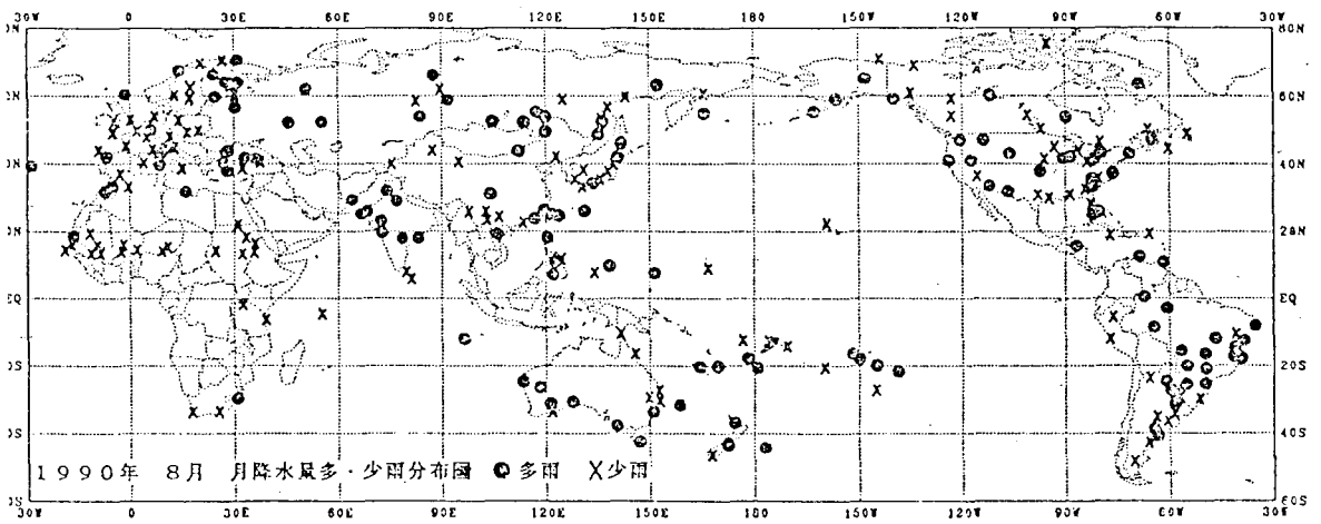
圖3.8 1990年8月月降水量多、少分布圖
