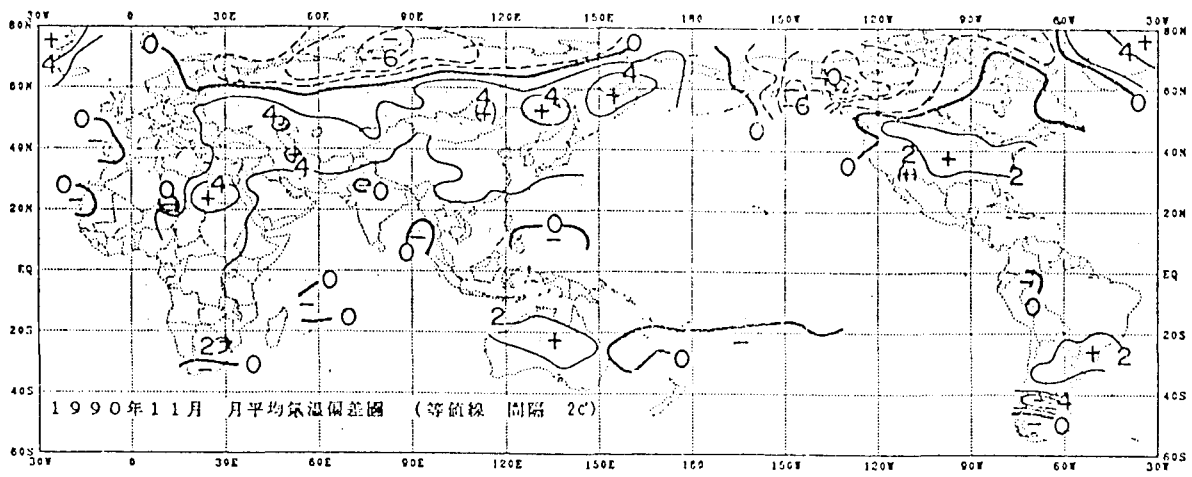
圖2.11 1990年11月月平均氣溫偏差圖
