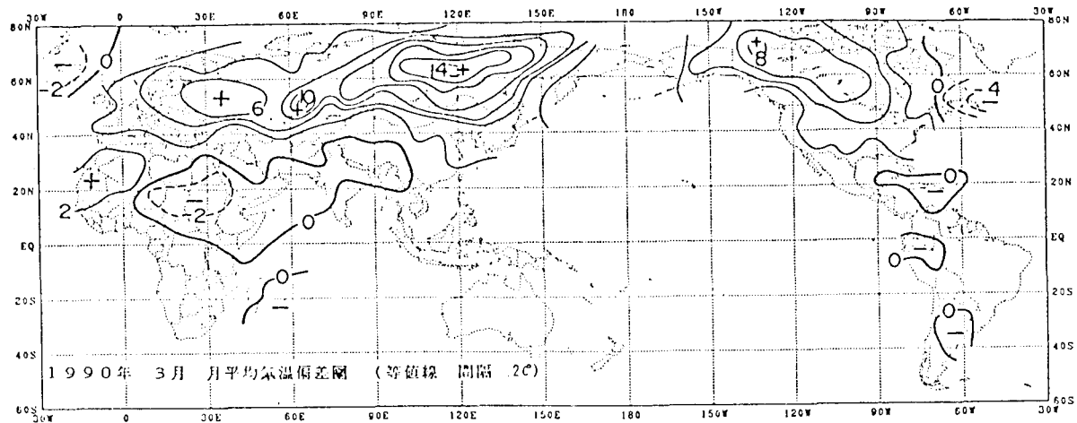
圖2.3 1990年3月月平均氣溫偏差圖
