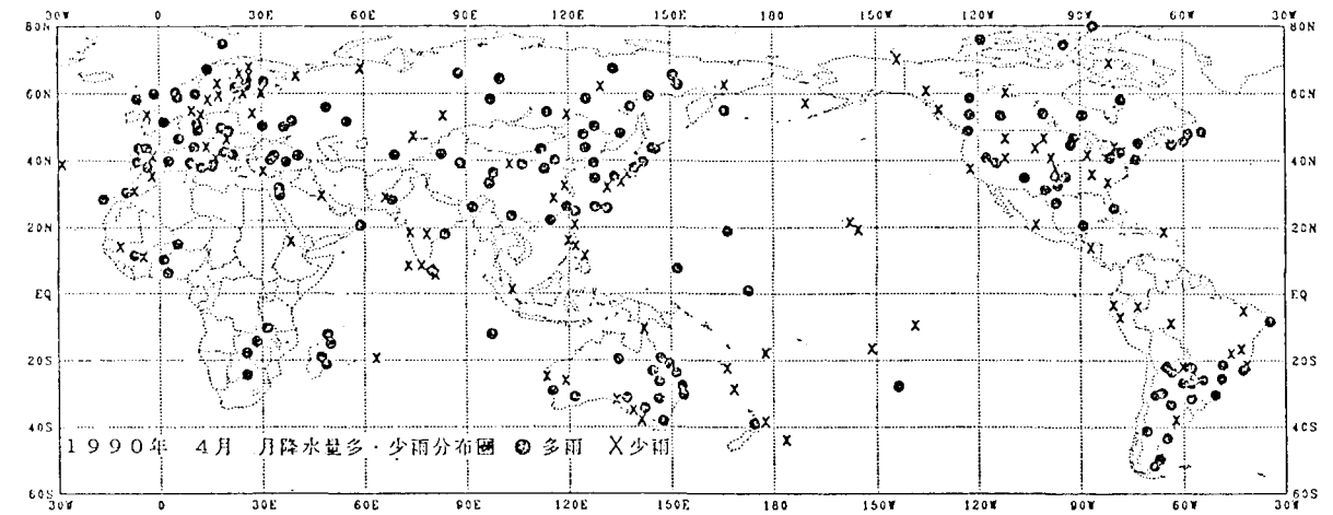
圖3.4 1990年4月月降水量多、少分布圖
