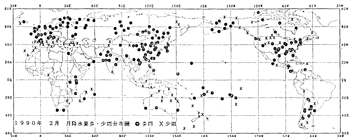
圖3.2 1990年2月月降水量多、少分布圖
