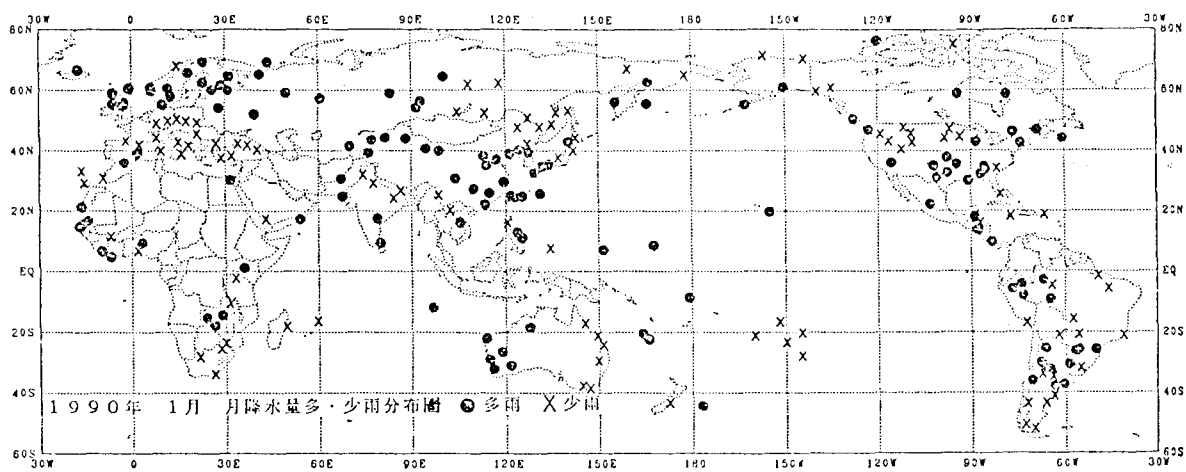
圖3.1 1990年1月月降水量多、少分布圖
