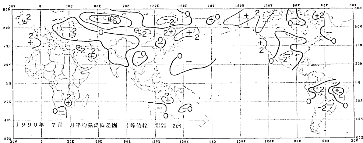
圖2.7 1990年7月月平均氣溫偏差圖
