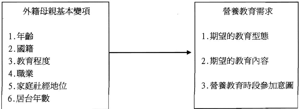
圖3-1 研究架構
