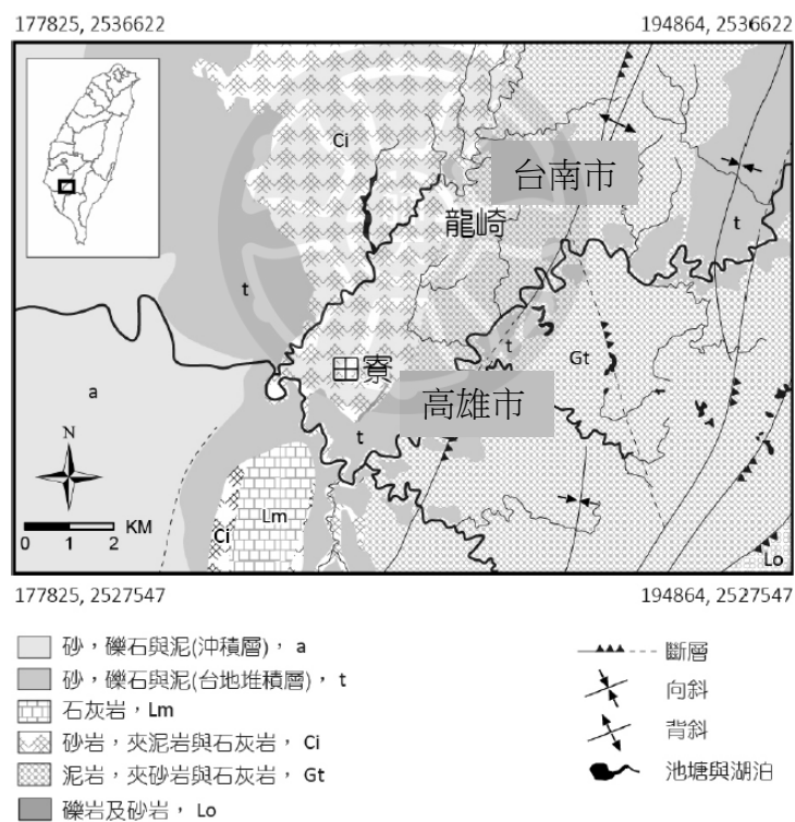
圖5 龍崎地區地質概況圖
