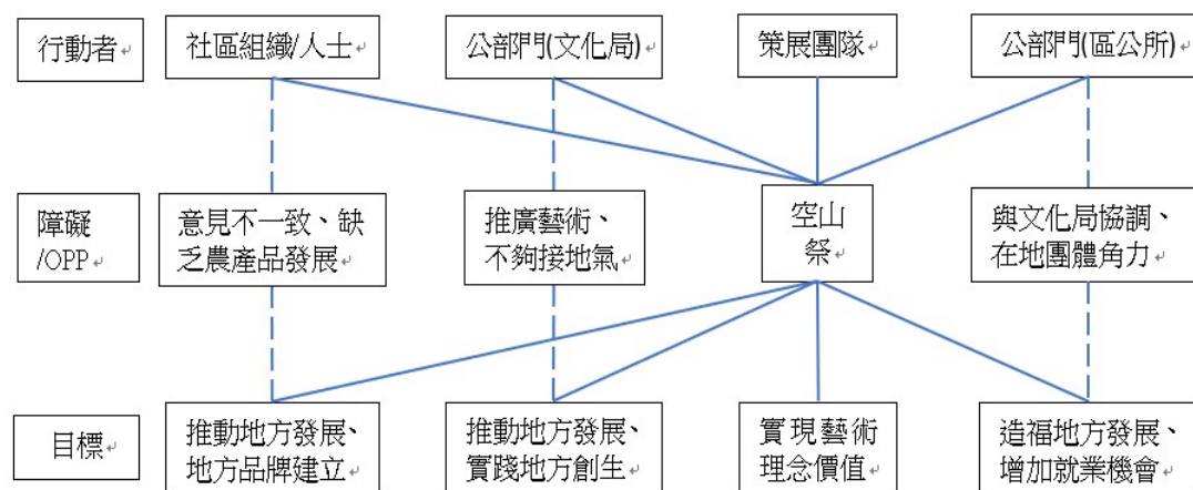
圖12 空山祭行動者網絡圖
